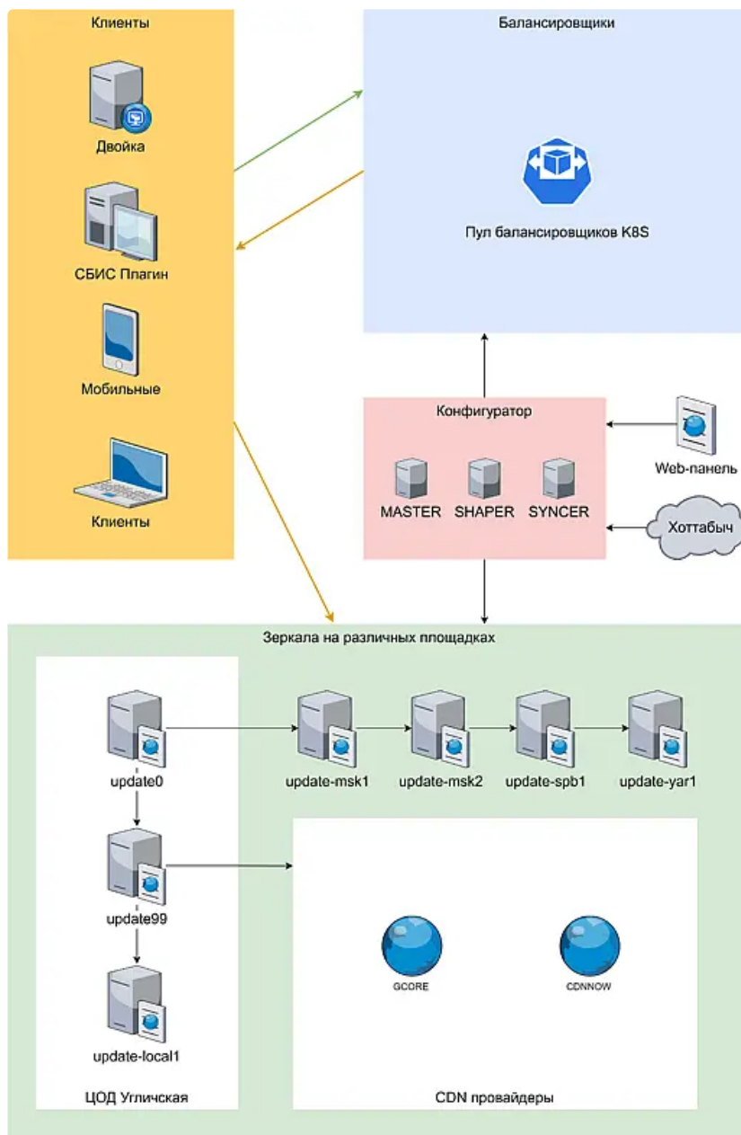
Рисунок 2. Схема архитектуры приложения
